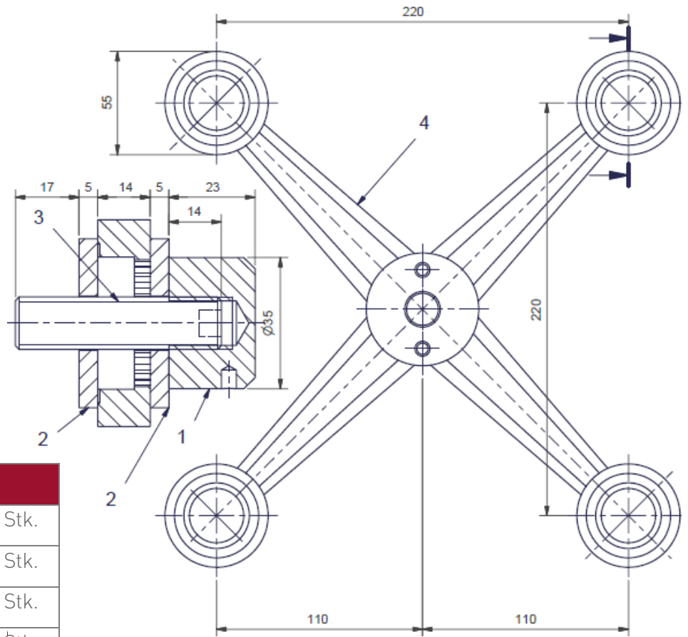
punktgehaltene, flächenbündige Glasbefestigung
