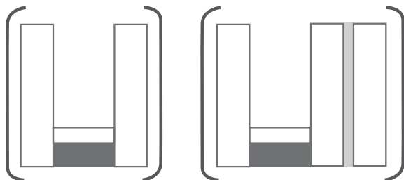
Abb. 31: Bsp. Einheit für Zweifachisolierverglasung
